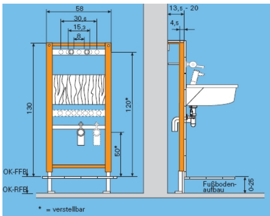
101 850 SanTec FIX výlevka
